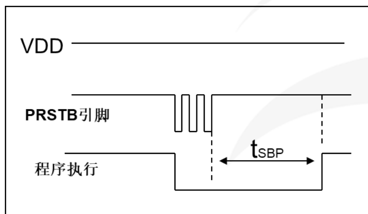
图 12：外部引脚复位的相关时序
