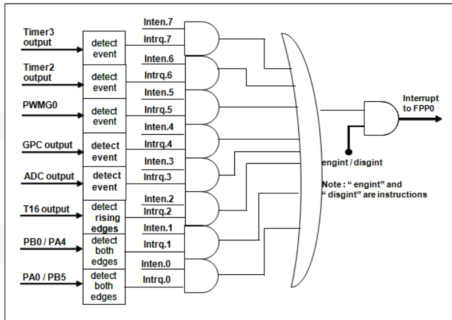
图 13: 中断硬件框图
