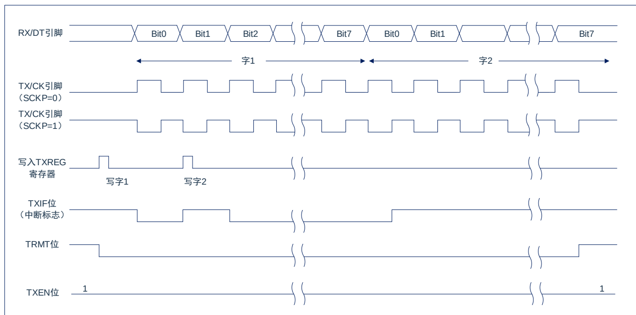
图 16-6：同步发送
