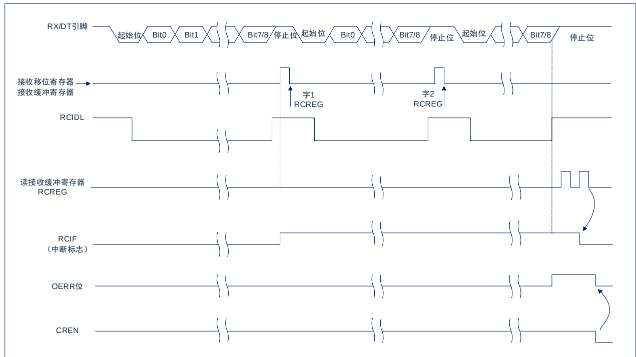
图 16-5: 异步接收
