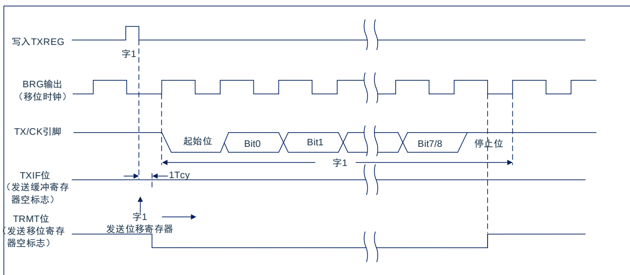
图 16-3: 异步发送
